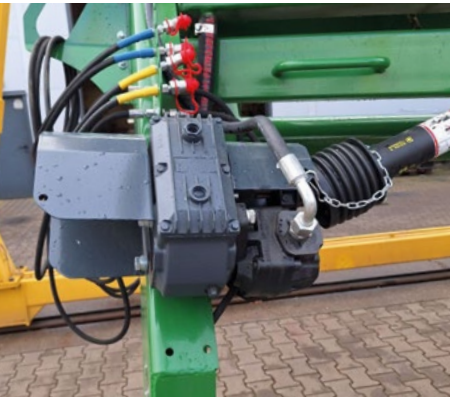
Autonominė tepalo sistema ant ZRM-180. Užtikrina tolygų tepalo padavimą į hidrovarklius
