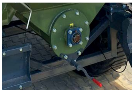
Винтов механизъм за отваряне на капаците за почистване на хоризонталния шнек
