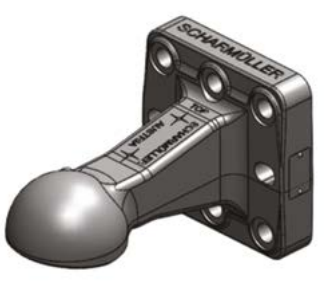
hemisphere Ø80
